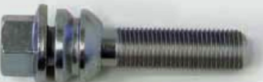
KUGELBUNDSCHRAUBEN Ø 28 MM MIT BEWEGLICHEM KUGELBUND, SW 19 (FÜR PORSCHE CAYENNE, VW TS, VW TOUAREG) / BOULONS À TÊTE SPHÉRIQUE Ø 28 MM AVEC SPHÈRE MOBILE, T 19 (POUR PORSCHE CAYENNE, VW TS, VW TOUAREG)
